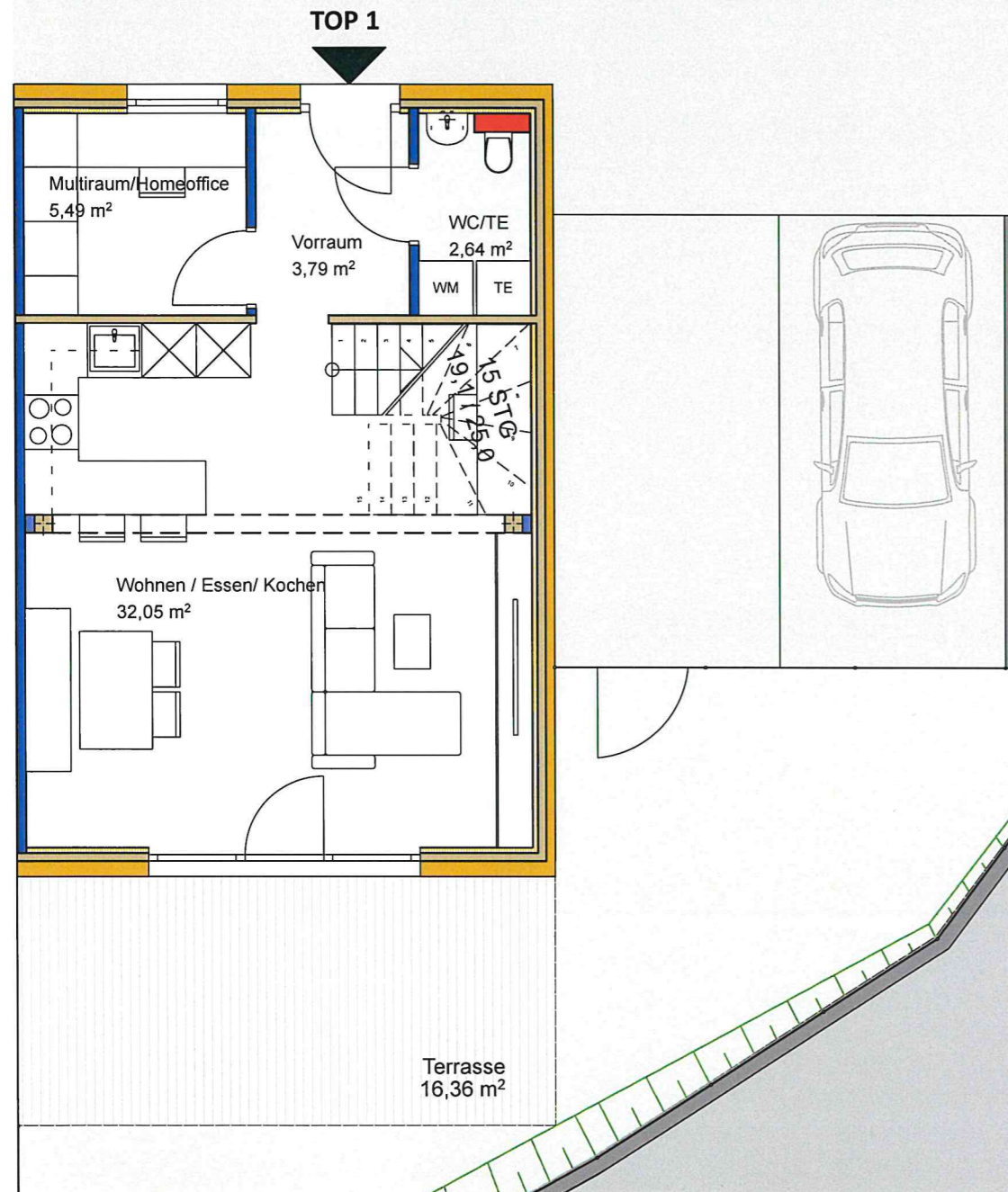
ERDGESCHOSS
