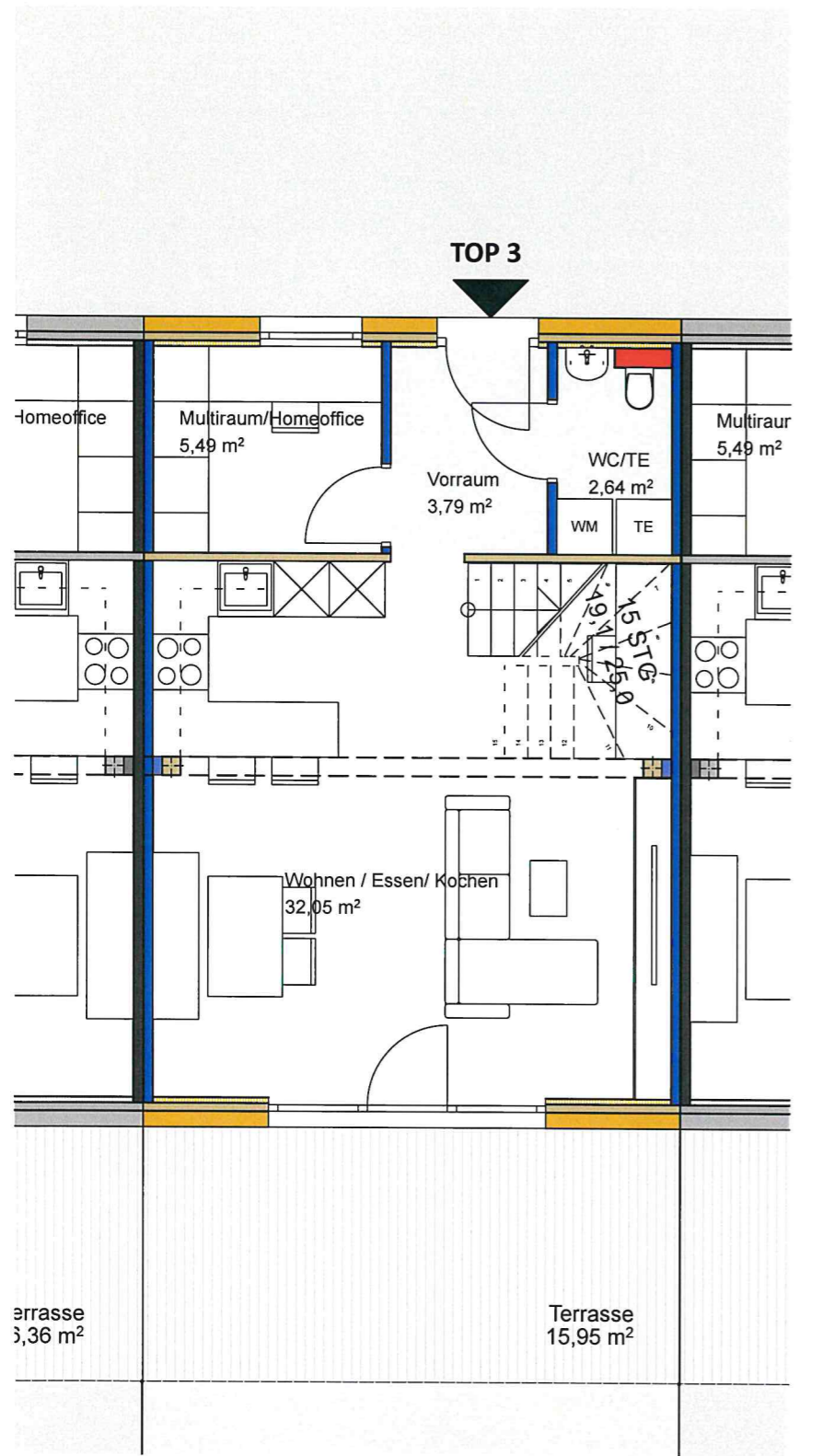
ERDGESCHOSS
